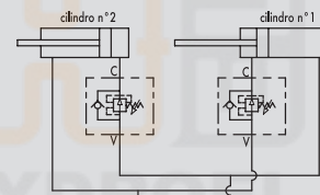
SCHEMA DI MONTAGGIO APPLICATION SCHEME
